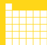
Verbleibendes Budget Deutschland für 1,5 Grad Ziel (3,1 Gigatonnen)
