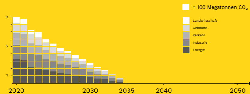
CO 2 -Emissionen nach Planung von GermanZero
