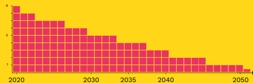
CO 2 -Emissionen nach Planung der Bundesregierung
